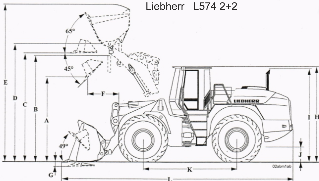
Abmessungen – Ausführung mit kurzem Z-Hubgerüst
